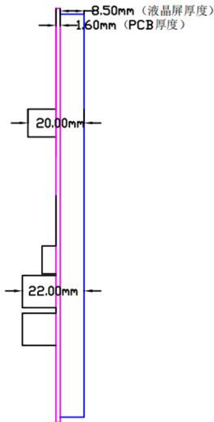
左侧面图
